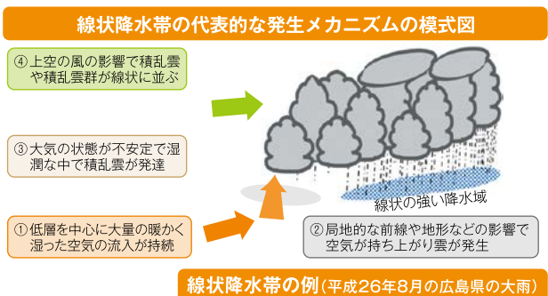
線状降水帯の例(平成26年8月の広島県の大雨)
